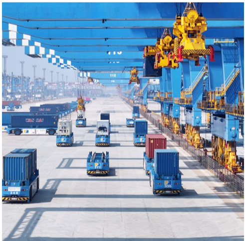
在自动化码头,AGV自动导引车正有序进行集装箱装卸作业。
