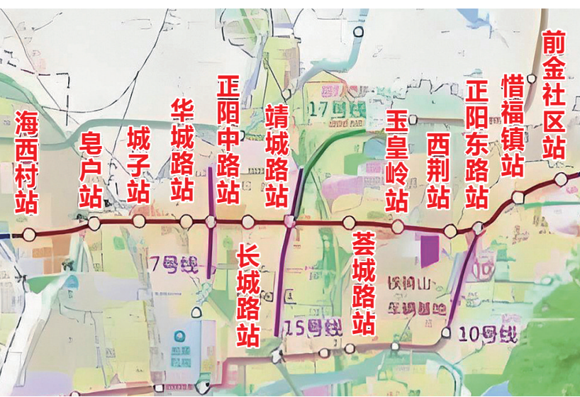
青岛地铁 9 号线一期线路示意图。青岛地铁供图
