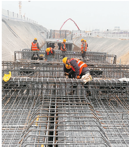
合肥路市政配套工程施工现场。
