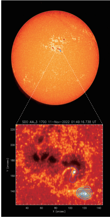
左图:“夸父一号”卫星HXI载荷对太阳耀斑的两能段硬X射线成像(25-30和30-35 keV,等值线)叠加在SDO卫星AIA 1700 图像背景上。
