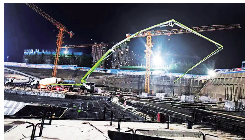
首块筏板顺利浇筑。
