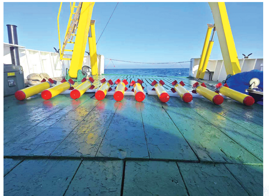
■空投型快速自动剖面浮标南海海试现场。
