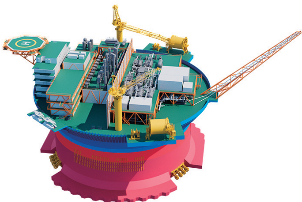
■开平南油田开发项目圆筒型浮式生产储卸油装置效果图。
