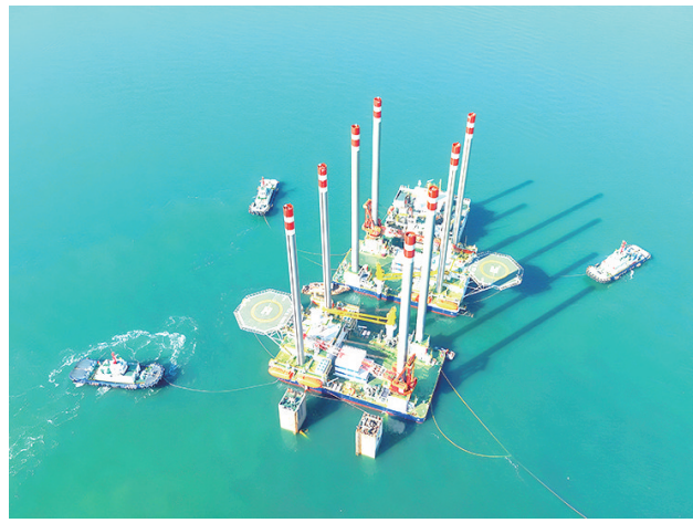
■海西重机两座TYPE3 PRO型自升式海上作业支持平台从青岛启航。
