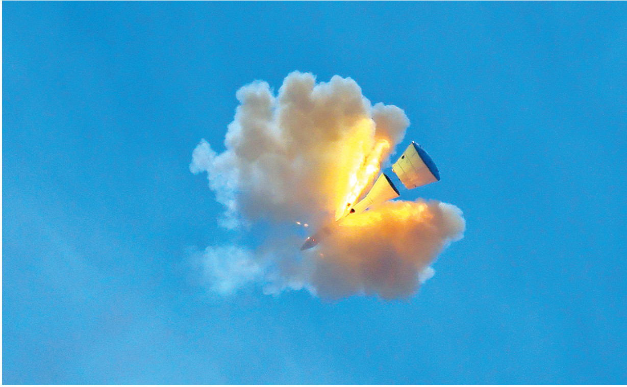
■6月17日，我国在酒泉卫星发射中心成功组织实施梦舟载人飞船零高度逃逸飞行试验，标志着我国载人月球探测工程研制工作取得新的重要突破。新华社照片
