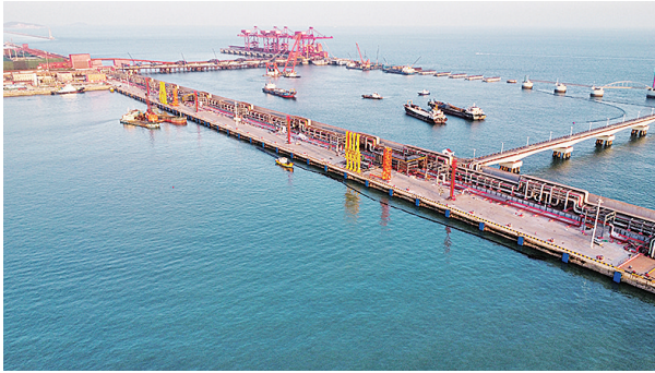
建成投产的青岛港董家口港区12万吨级油品码头工程。
