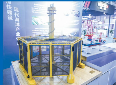
■“深蓝1号”网箱模型。
