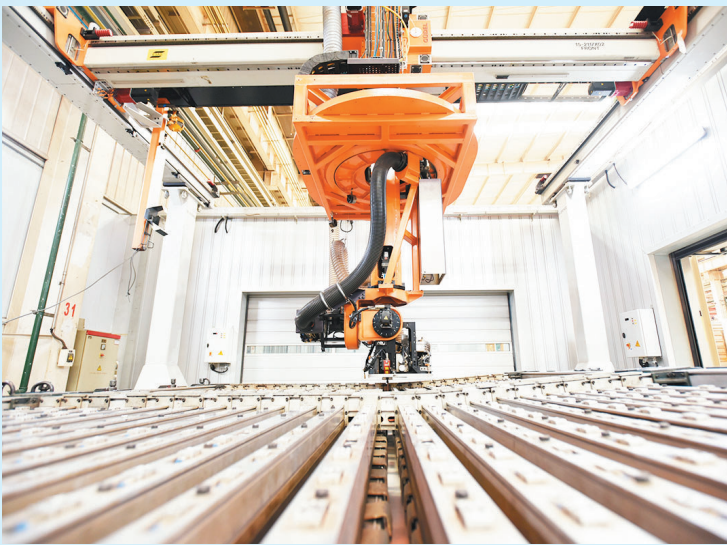
■中车四方股份公司高速动车组数字化焊接生产线。
