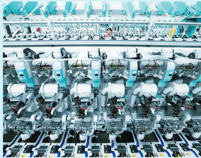
■即发10万纱锭数字化纺纱智能工厂。
