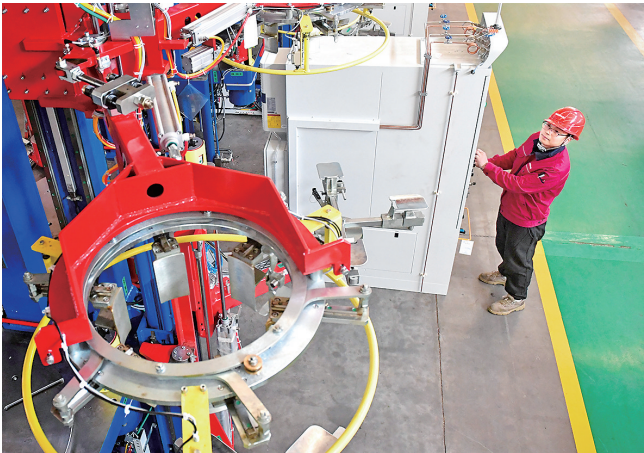
■在软控装备产业园，技术员张文建正在精心调试智能化轮胎硫化设备。 赵健鹏 摄
