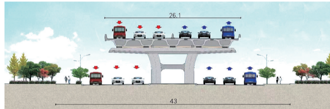
高架标准段横断面示意图。
